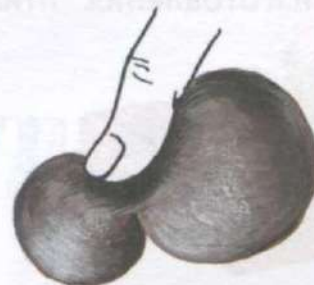
Примазывание
